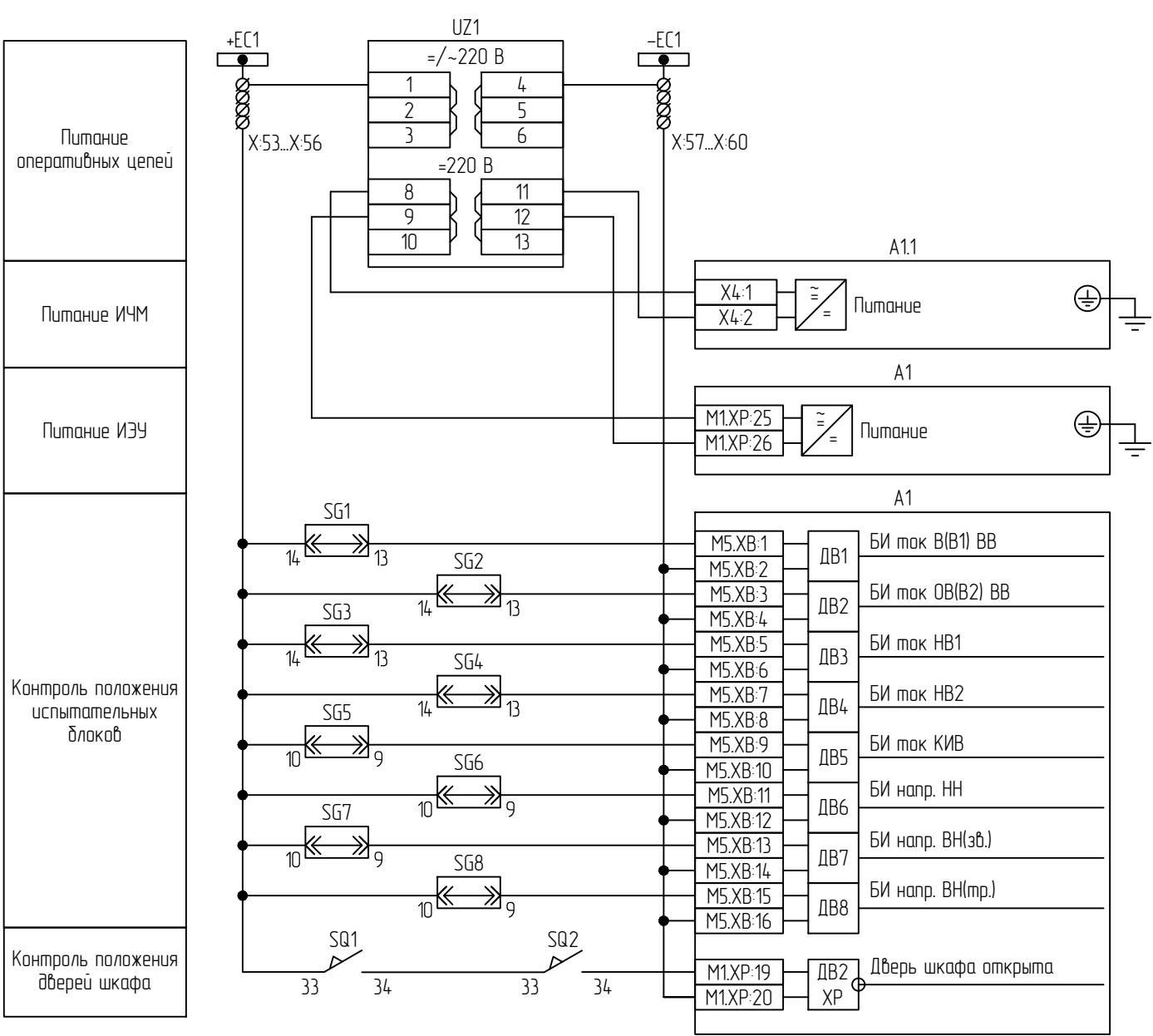
Цепи оперативного тока
